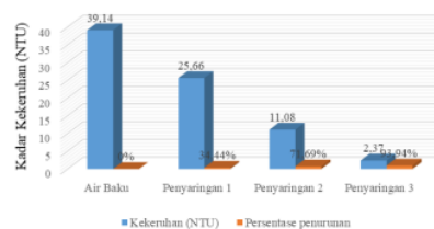
Gambar 2. Hasil Penurunan Kekeruhan
