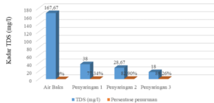
Gambar 3. Hasil Penurunan TDS
