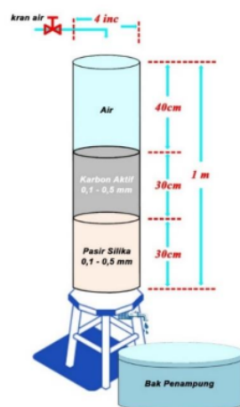
Gambar 1. Alat Filtrasi Sederhana
